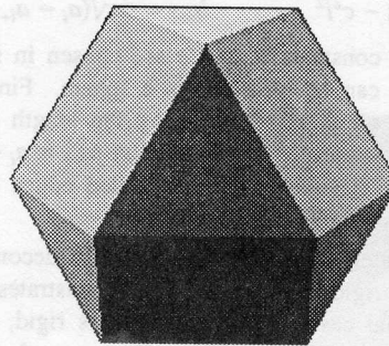
Fig. 2. A cubo-octahedron.
