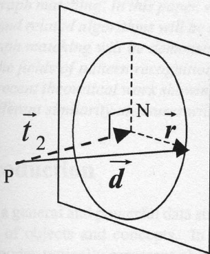
Figure 9 : Redirection de \vec{t}_2 dans le plan orthogonal.
