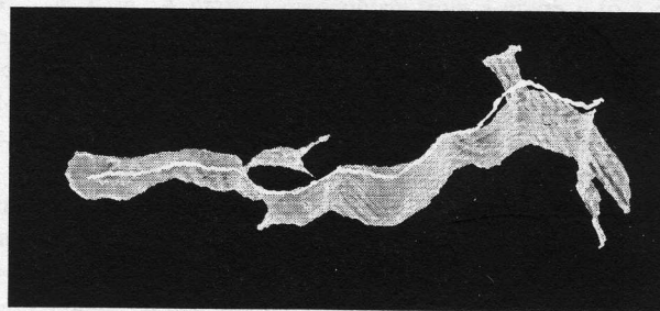
Figure 11 : En clair, le suivi correspondant au fond du sillon supérieur frontal.
