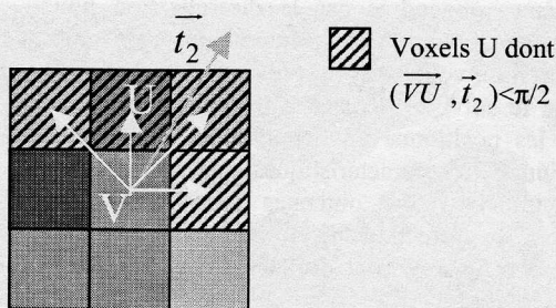
Figure 5 : Exemple en 2D du choix de la direction de propagation du suivi discret selon le cas 2. Le niveau de gris symbolise le niveau de courbure du voxel. Les valeurs de courbures fortes correspondent aux couleurs sombres.
