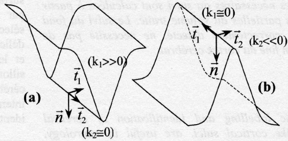
Figure 2 : (a) Vecteurs courbures principaux sur sillons, (b) Vecteur courbures principaux sur gyri.
