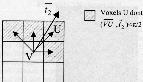
Figure 4 : Exemple en 2D du choix de la direction de propagation du suivi discret selon le cas 1
