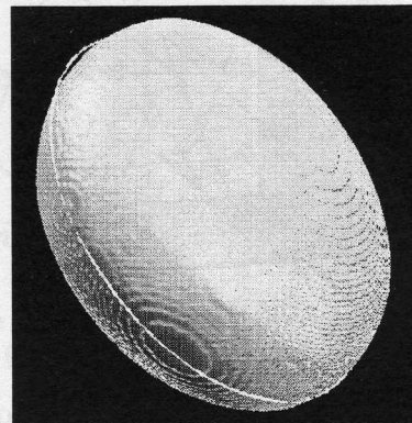
Figure 8 : En clair, ligne correspondant au suivi effectué sur l'ellipsoïde.
